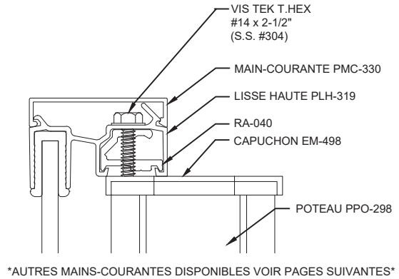
○ DÉTAIL A VUE 1:2
